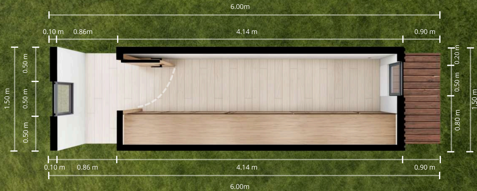
Vista en Planta de Walking closet
