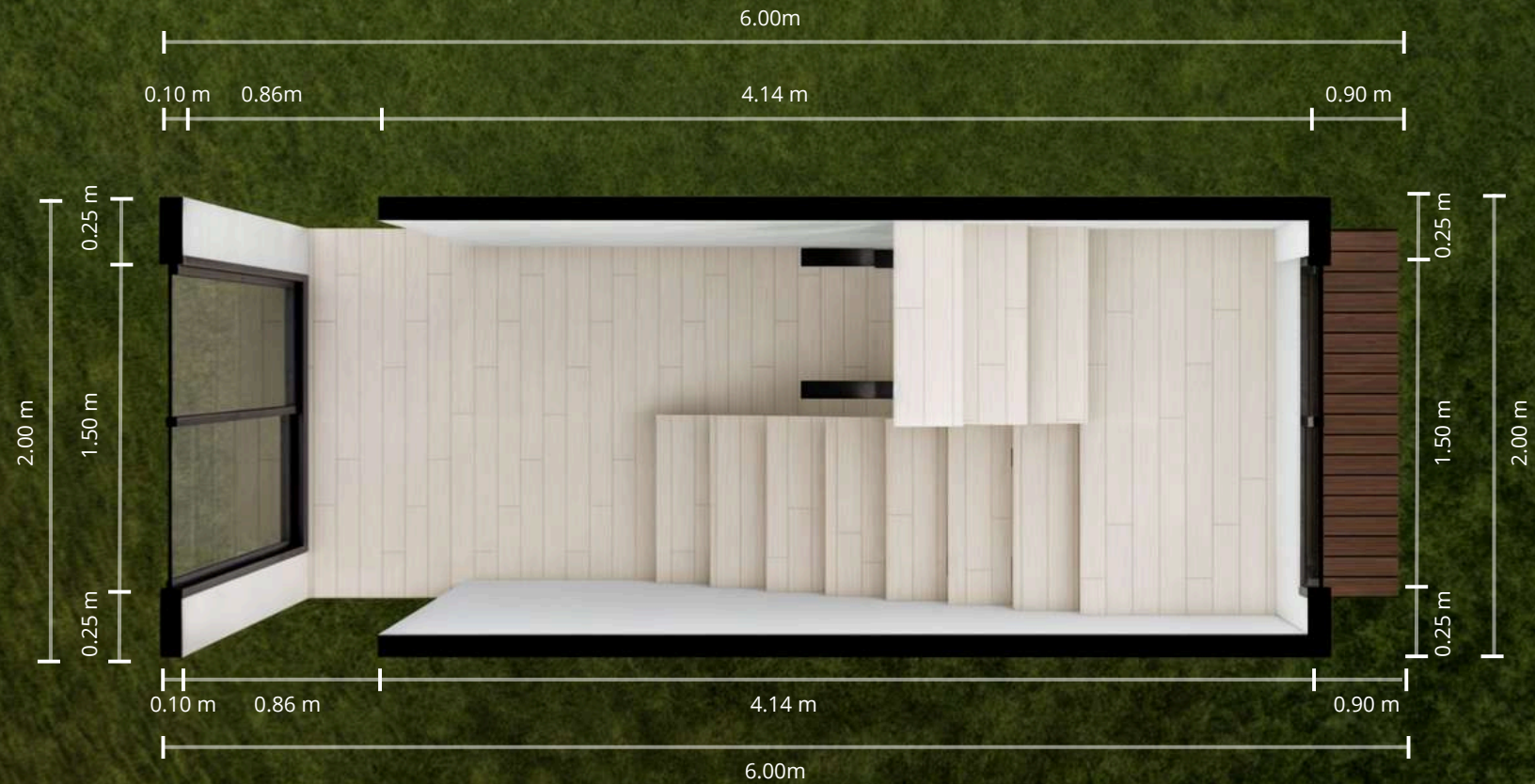
Vista en Planta Escalera
